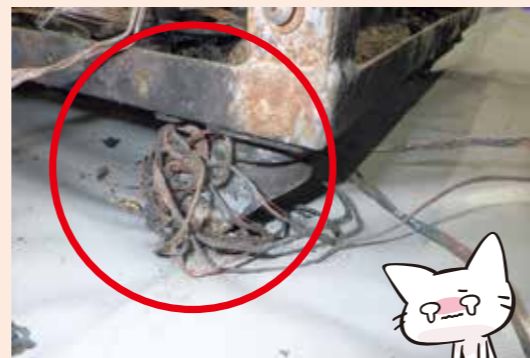
配線が原因で火災が生じた事例の写真。○の部分に配線の絡まりがあり、ここから出火しました。
